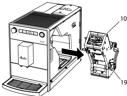
Afb. 12: Zetgroep demonteren
