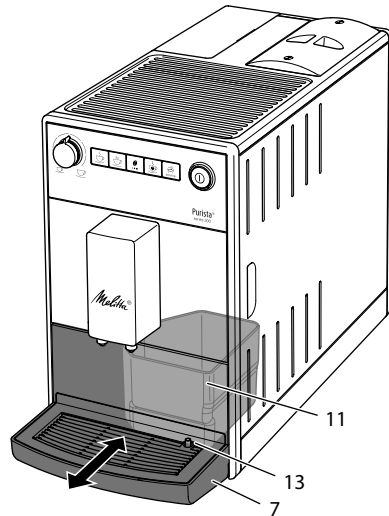
Abb. 8: Tropfschale und Kaffeersatzbehälter entleeren
