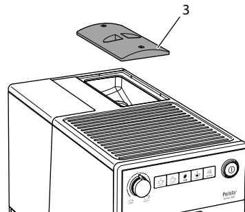
Pav. 5: Pupelių talpyklos dangtelio atvėrimas
